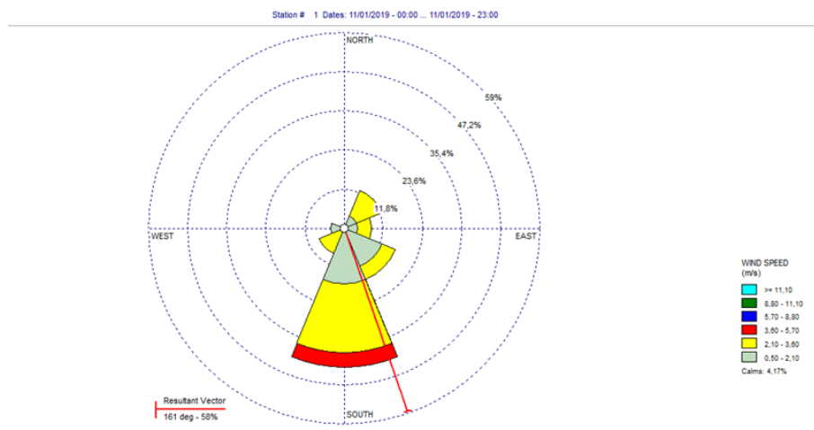
Figura 4. Rosa de Viento estación meteorológica UNICOMFACAUCA Fuente: Propia 2025
